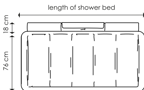
DIMENSIONS
